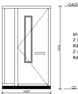
Merk: 20 2 st. getekend KAVEL 1, 3 2 st. gespiegeld KAVEL 2, 4
