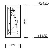
Merk: 11 (sp) 2 st. getekend KAVEL 1, 3 2 st. gespiegeld KAVEL 2, 4
