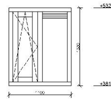
Merk: 07 2 st. getekend KAVEL 2, 4
