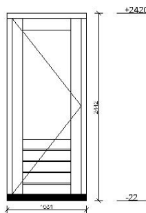
Merk: 12 (sp) 2 st. getekend / 2 st. gespiegeld KAVEL 1, 3, / 2, 4
